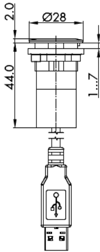
USB VCP
